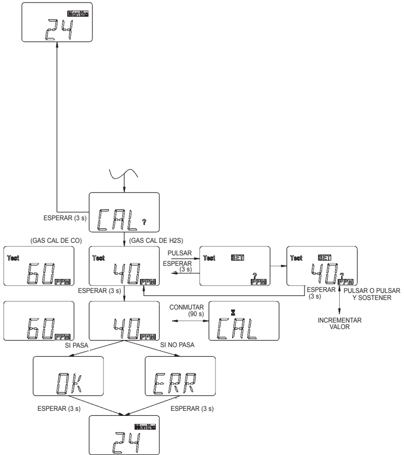
Figura 4-1. Diagrama de flujo de la calibración (de gases tóxicos) (parte 2 de 2)
